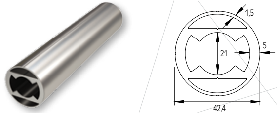
F50-107 Κολώνα Ø42 ενισχυμένη
