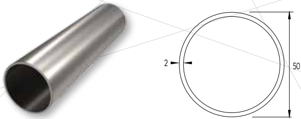
F50-200 Κουπαστή Ø50
