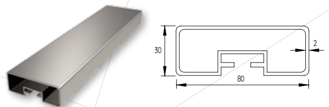
F50-201 Κουπαστή 30x80
